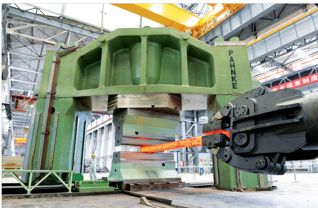
作业中的宝钛集团万吨自由锻压机
