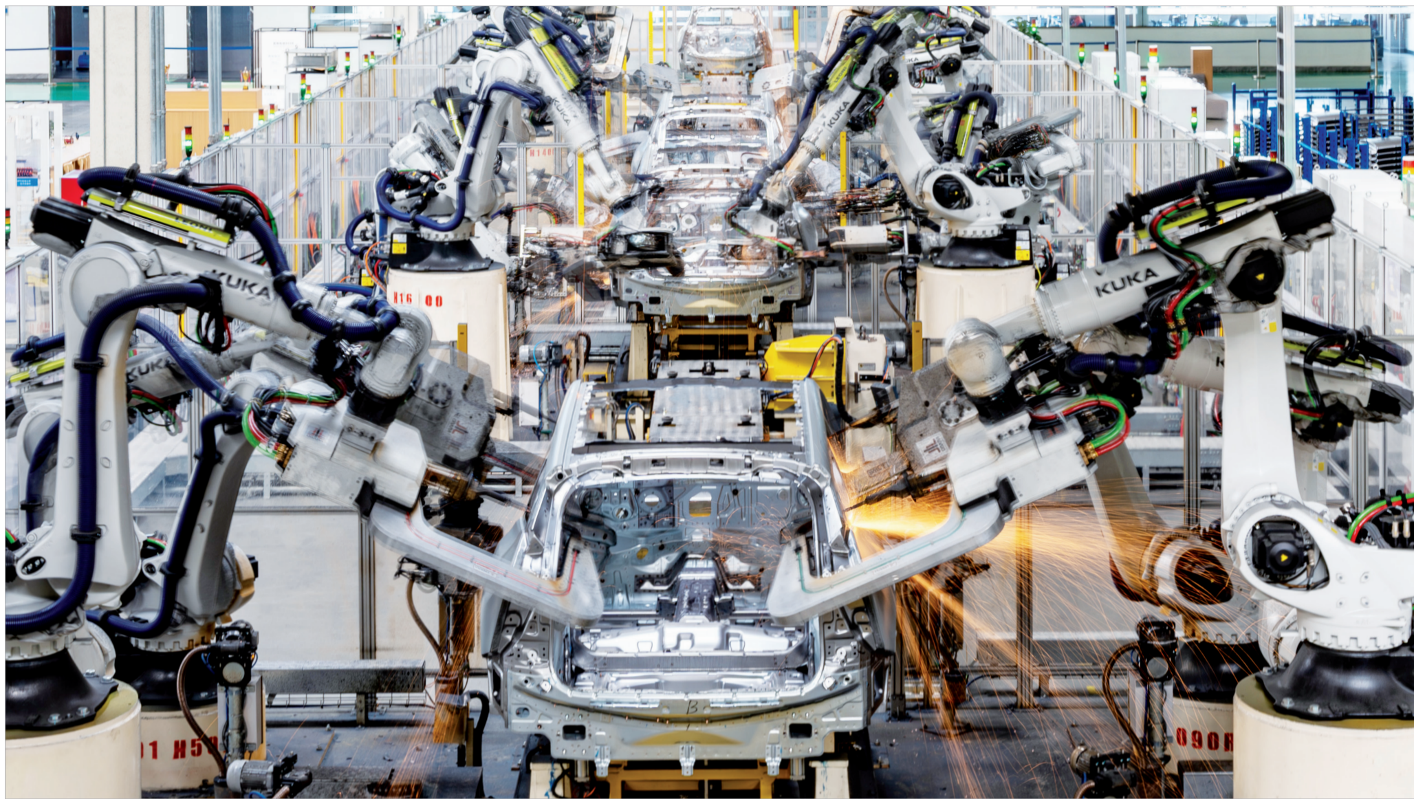
在吉利汽车宝鸡工厂，焊接、搬运、涂胶等实现了自动化。
