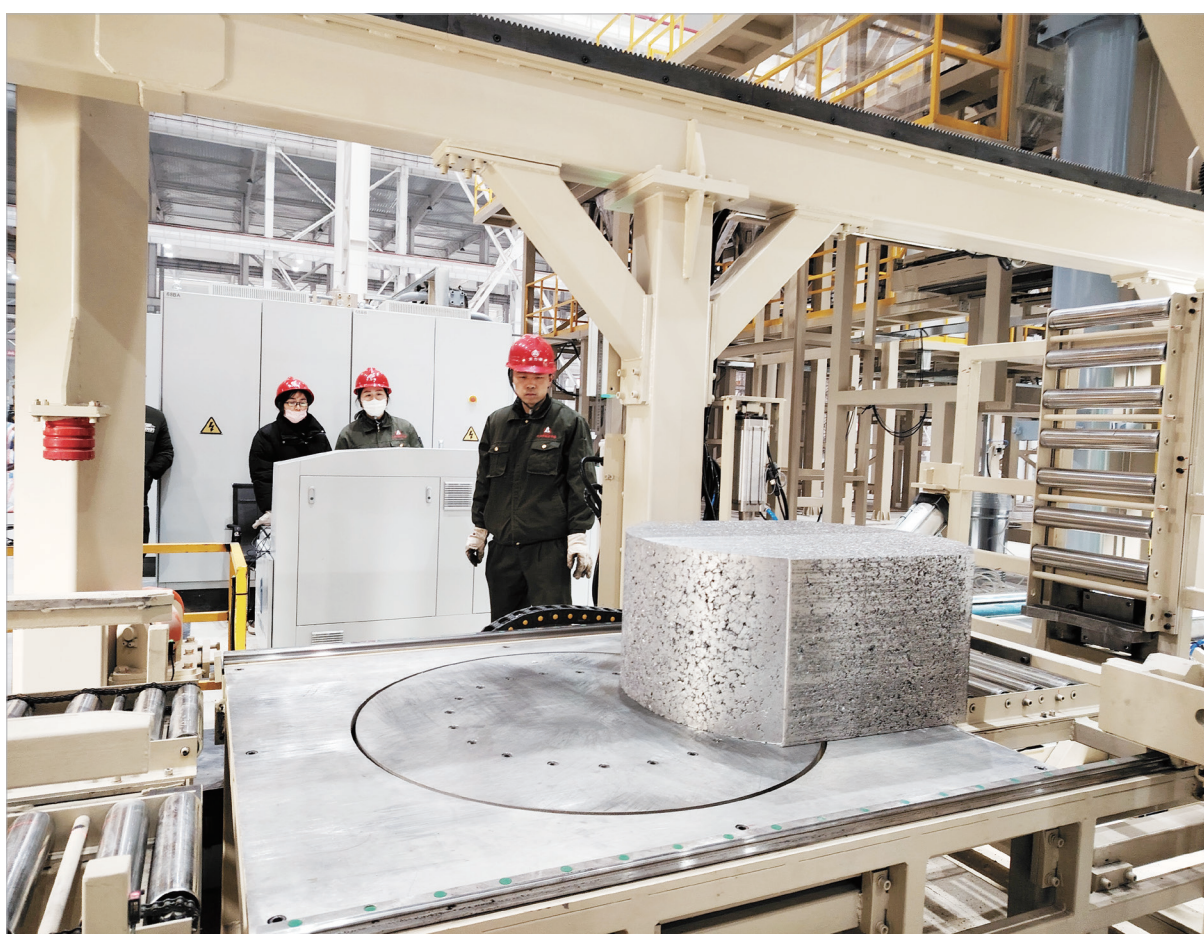
工人查看压制好的电极块
