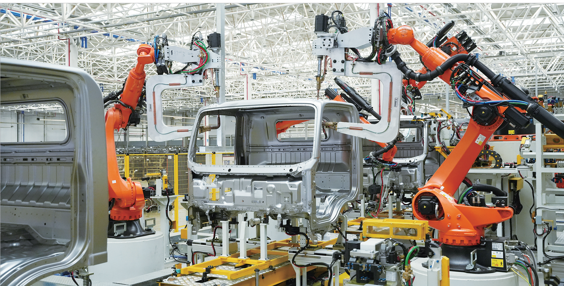
陕汽轻卡新平台焊接线
