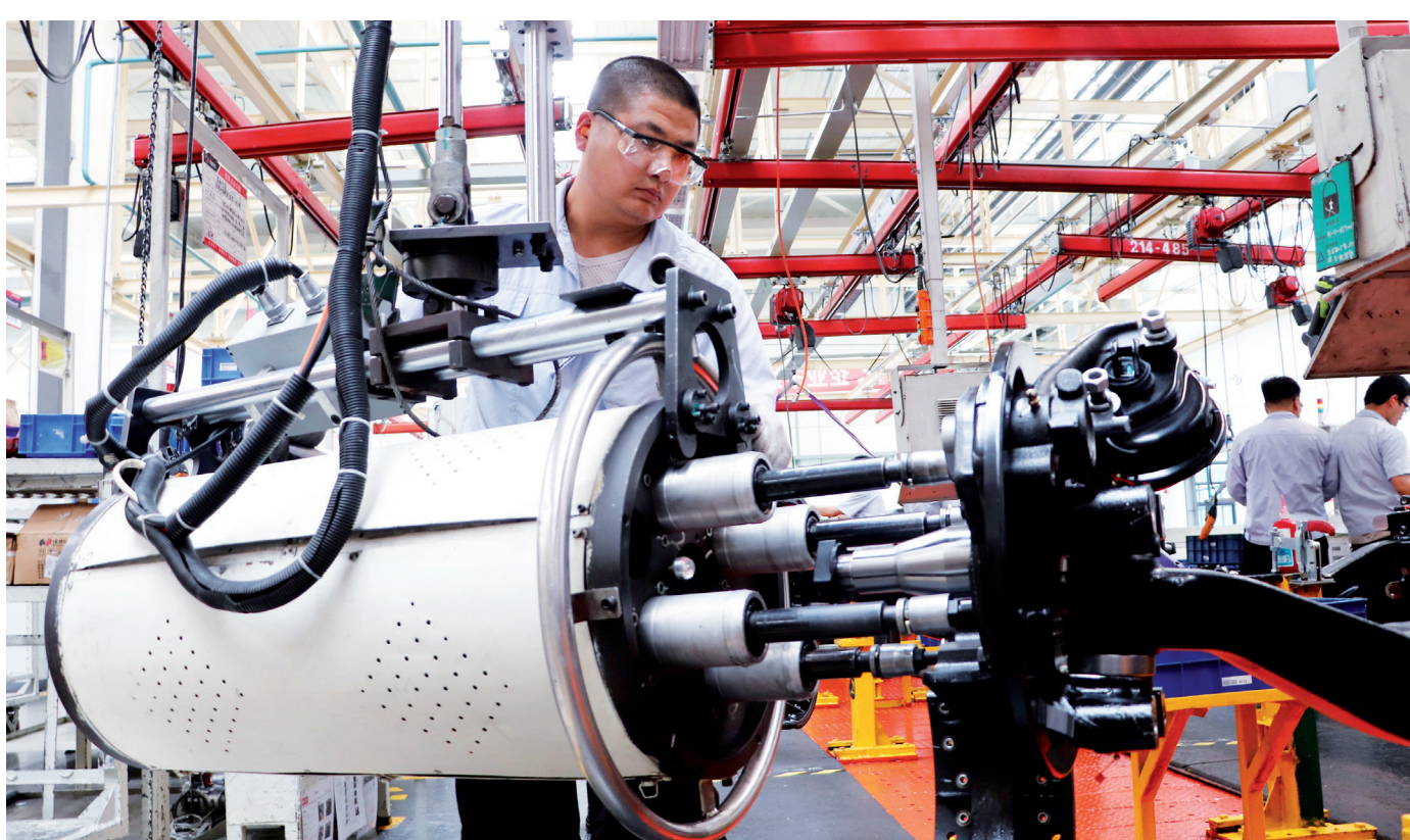
工人在组装车桥
