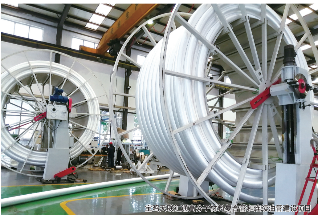
陕西中创精密传感技术有限公司生产车间
